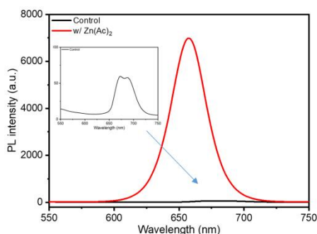
图 2 钙钛矿薄膜 PL 表征
