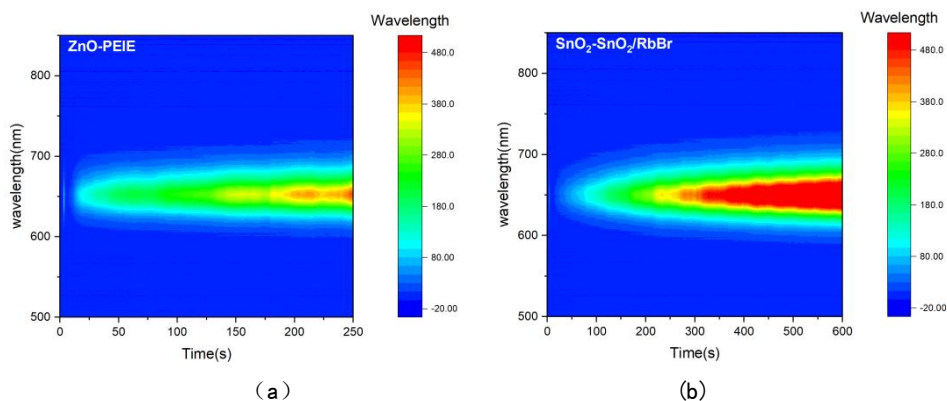
图 4 两种基底上钙钛矿薄膜原位退火 PL 表征: (a) ZnO 基底 (b) SnO 2 基底
