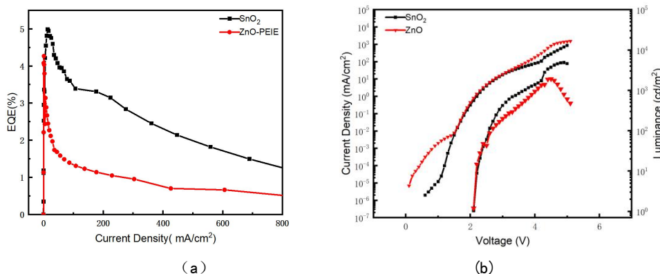
图 5 LED 器件性能表征: (a) 外量子效率; (b) 电流-电压-亮度曲线
