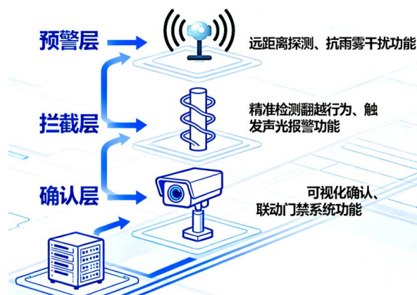
图 2 广州地铁车辆段分层周界安防架构图
