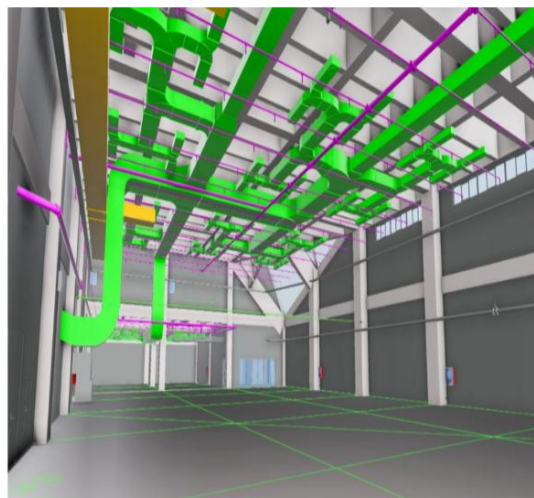
图 2: 管道设备定位与管道布置示意图
