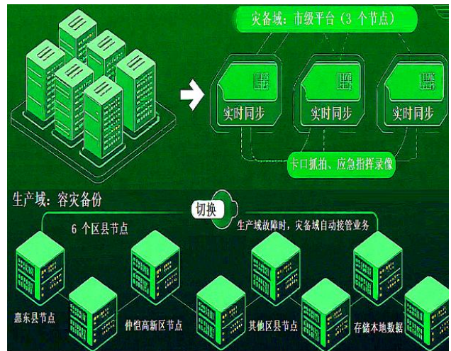
图 3：惠州“市级-区县级”容灾架构图
