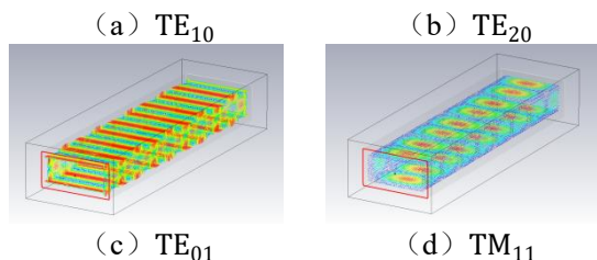
图 8 20GHz 下不同模式的表面电流
