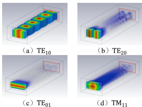
图 2 10GHz 下不同模式的导通状态
