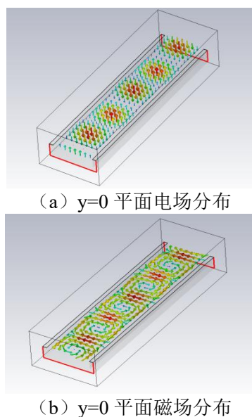
图 3 TE_{10} 模式 y=0 平面电场和磁场分布
