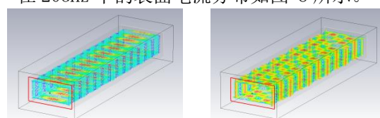
图 7 20GHz 下不同模式的导通状态
